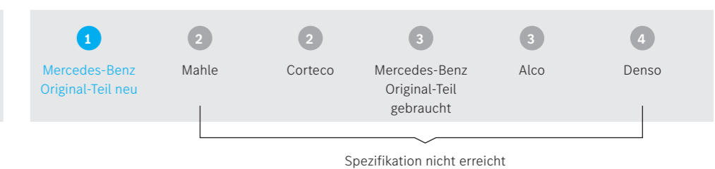
Ranking Fraktionsabscheidung
